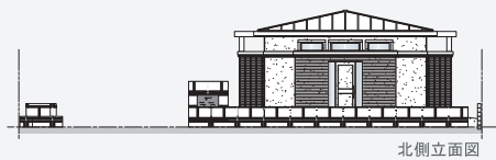
北側立面図
